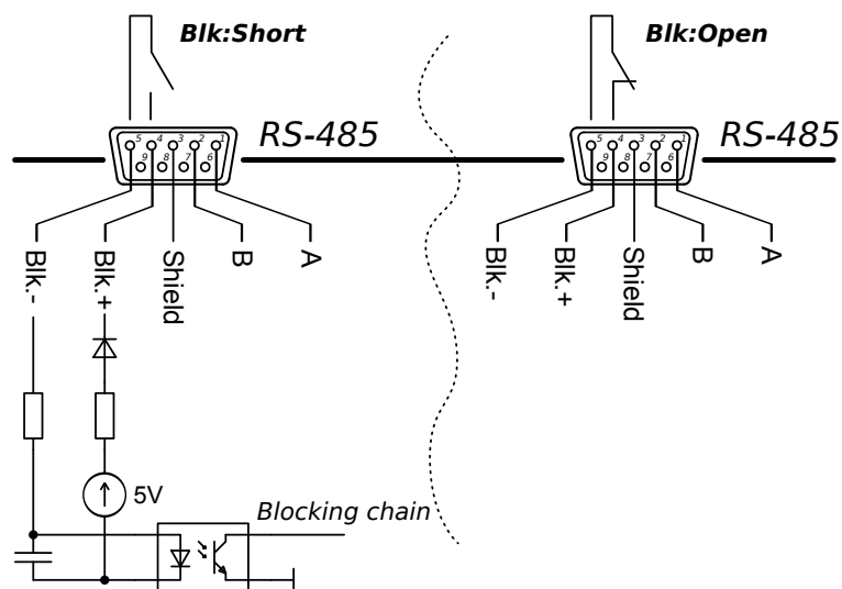
Рис. 1 — Схема цепи блокировки APEL-H-10DC-400.
