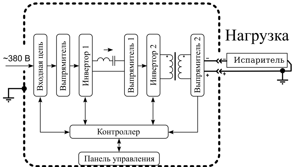
Рис. 1 — Структурная схема APEL-H-10DC-400.
