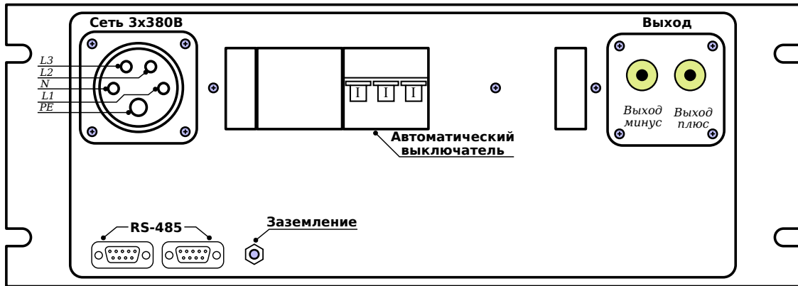
Рис. 3 — Задняя панель ИП APEL-H-10DC-400.
