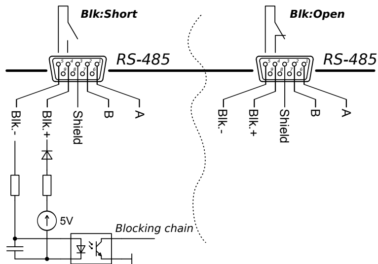
Рис. 1 — Схема цепи блокировки APEL-IS-3500-N.
