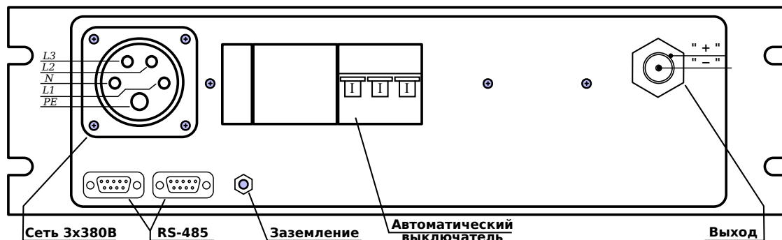
Рис. 3 — Задняя панель ИП APEL-IS-3500-N.
