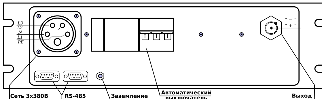
Рис. 3 — Задняя панель ИП APEL-IS-6000.
