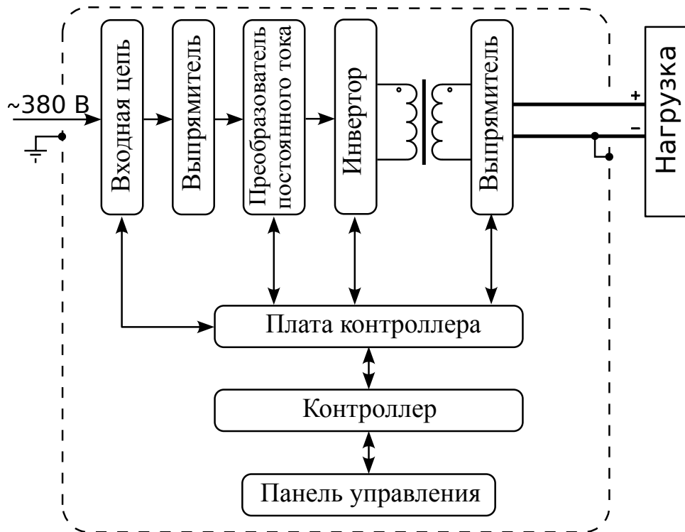
Рис. 1 — Структурная схема APEL-IS-6000.
