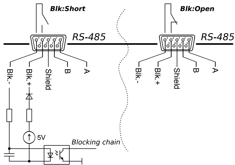
Рис. 1 — Схема цепи блокировки APEL-IS-6000.
