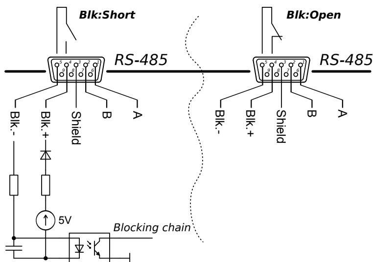
Рис. 1 — Схема цепи блокировки APEL-M-1.5BP-1000-1.
