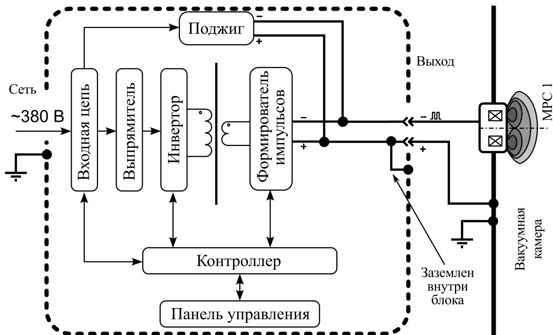
Рис. 1 — Структурная схема источника питания APEL-M-1.5BP-1000-1.
