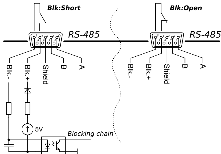
Рис. 1 — Схема цепи блокировки APEL-M-1.5BP-1000-2.
