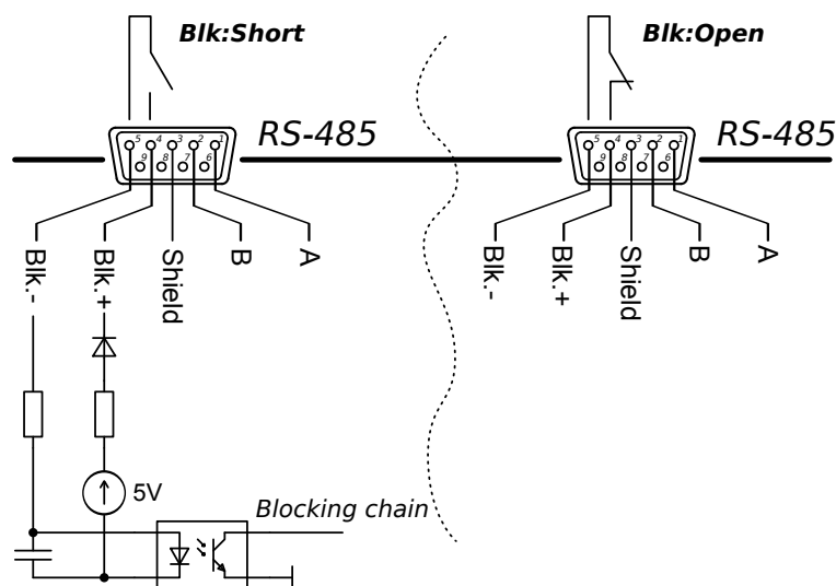
Рис. 1 — Схема цепи блокировки APEL-M-1.5BP-650-1.
