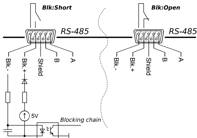
Рис. 1 — Схема цепи блокировки APEL-M-1.5BP-800-2.
