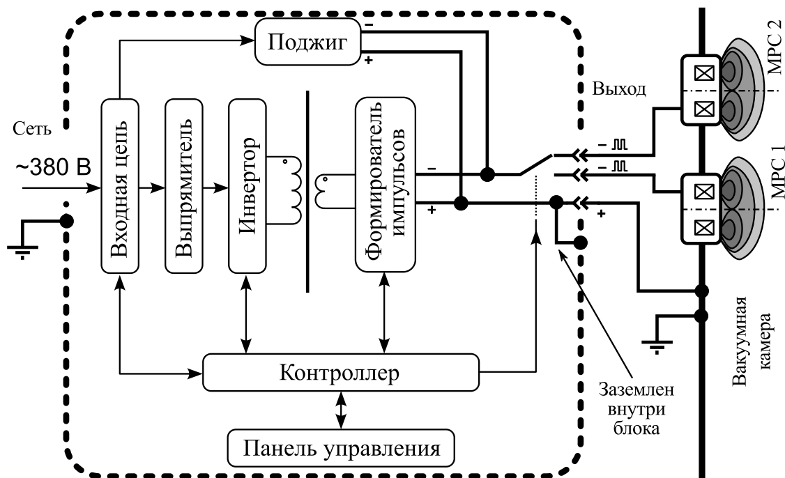
Рис. 1 — Структурная схема источника питания APEL-M-1.5BP-800-2.
