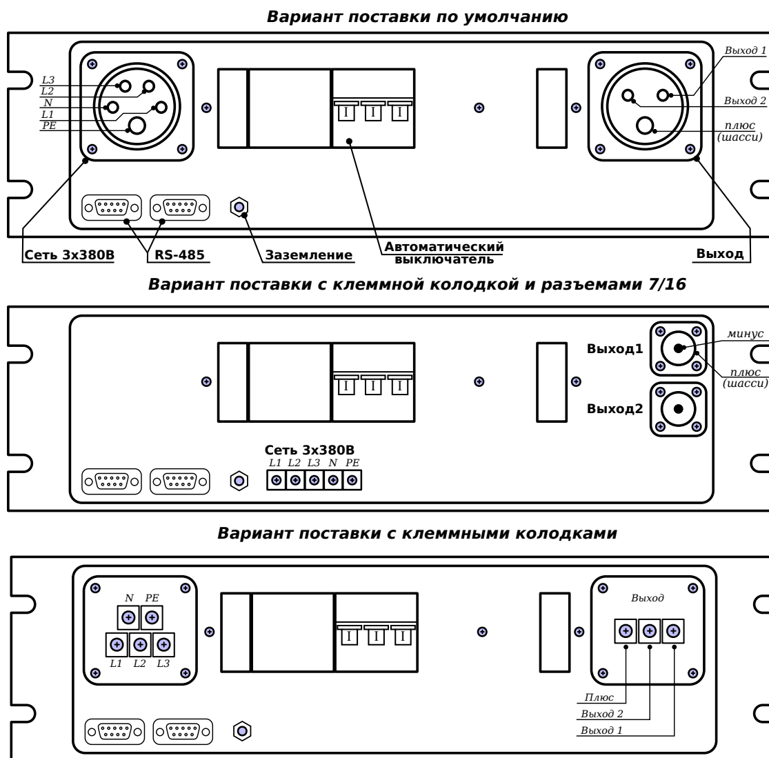
Рис. 3 — Задняя панель ИП APEL-M-1.5BP-800-2.
