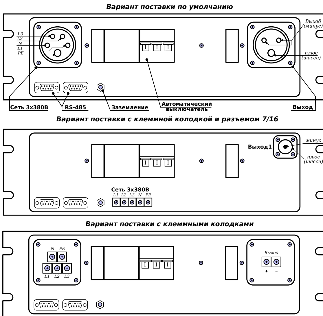
Рис. 3 — Задняя панель ИП APEL-M-1.5PDC-1000-1.
