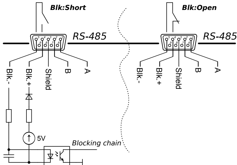
Рис. 1 — Схема цепи блокировки APEL-M-1.5PDC-1000-2.
