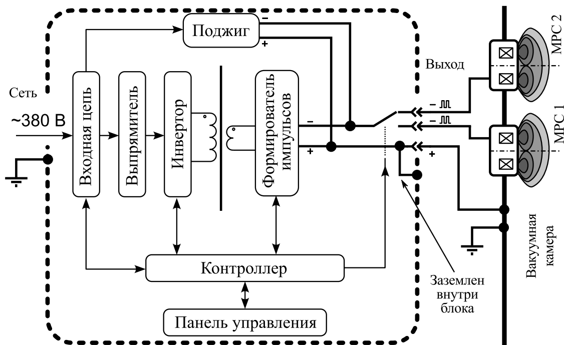
Рис. 1 — Структурная схема источника питания APEL-M-1.5PDC-1000-2.
