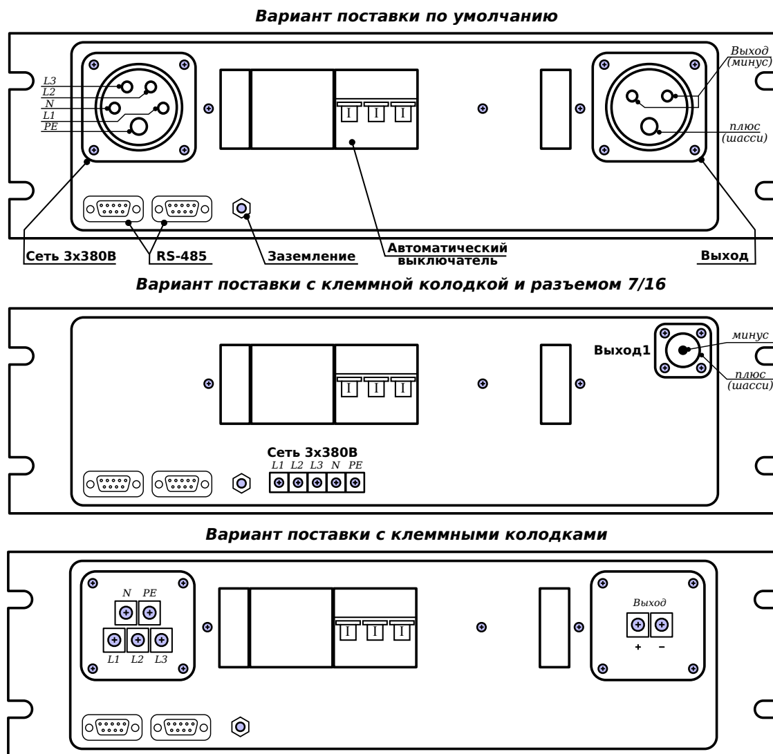
Рис. 3 — Задняя панель ИП APEL-M-1.5PDC-650-1.
