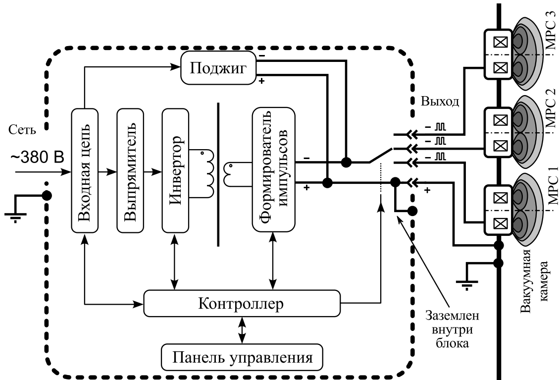
Рис. 1 — Структурная схема источника питания APEL-M-1.5PDC-650-3.
