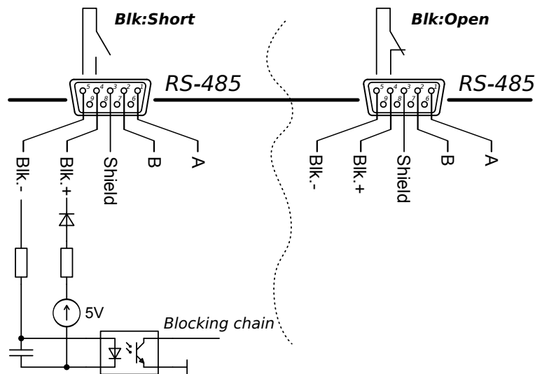
Рис. 1 — Схема цепи блокировки APEL-M-1.5PDC-650-3.
