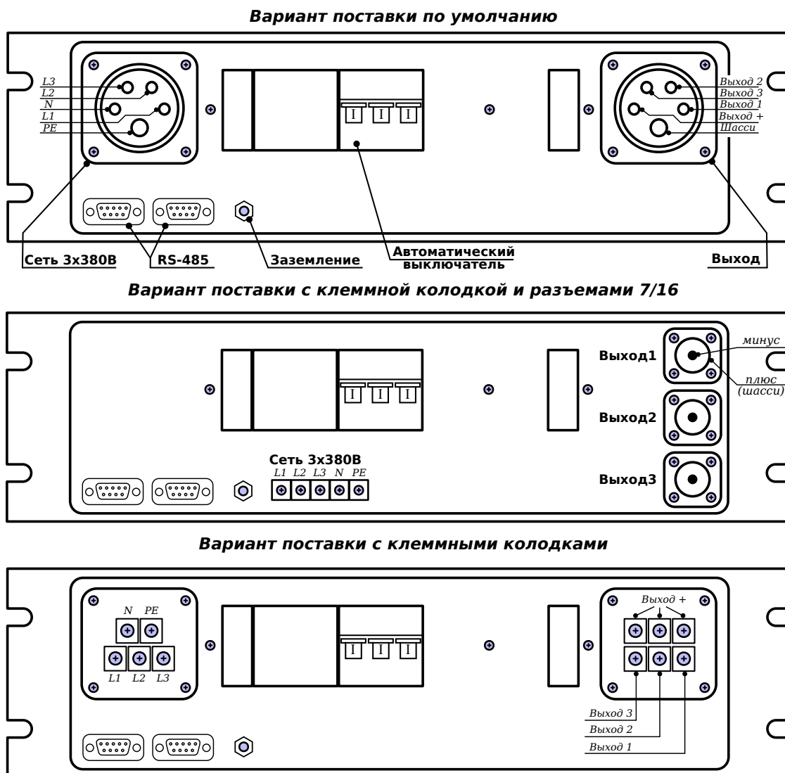
Рис. 3 — Задняя панель ИП APEL-M-1.5PDC-650-3.
