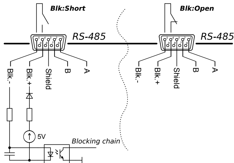
Рис. 1 — Схема цепи блокировки APEL-M-1.5PDC-800-1.
