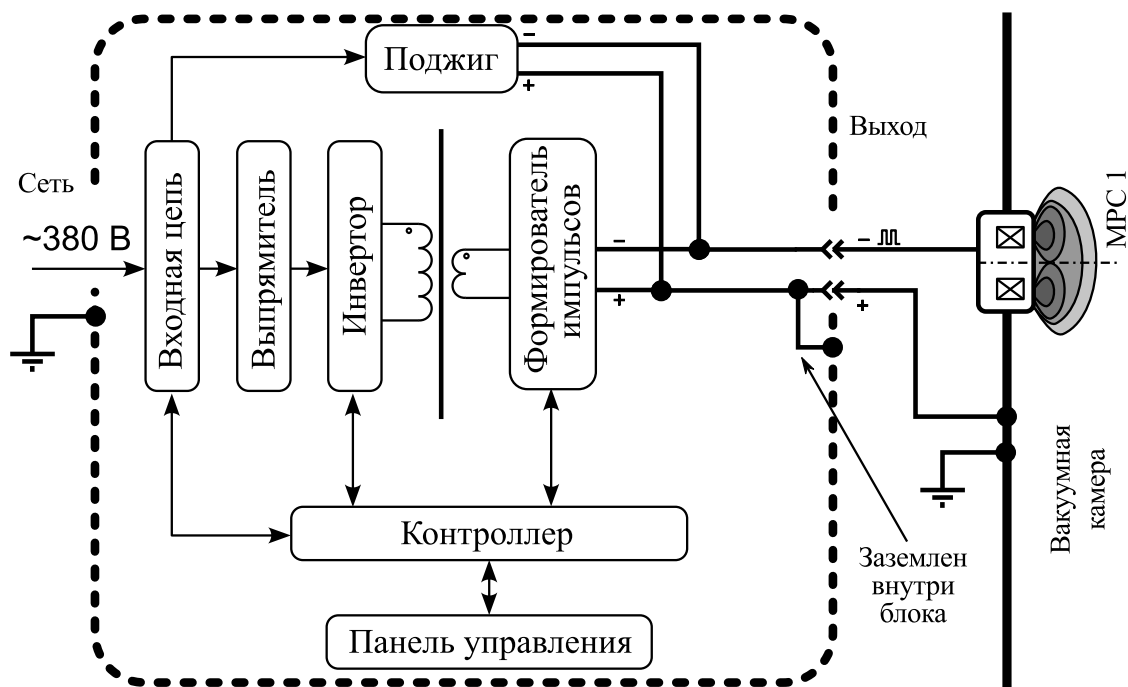
Рис. 1 — Структурная схема источника питания APEL-M-1.5PDC-800-1.
