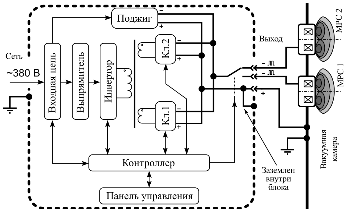
Рис. 1 — Структурная схема источника питания APEL-M-10BP-1000-2.
