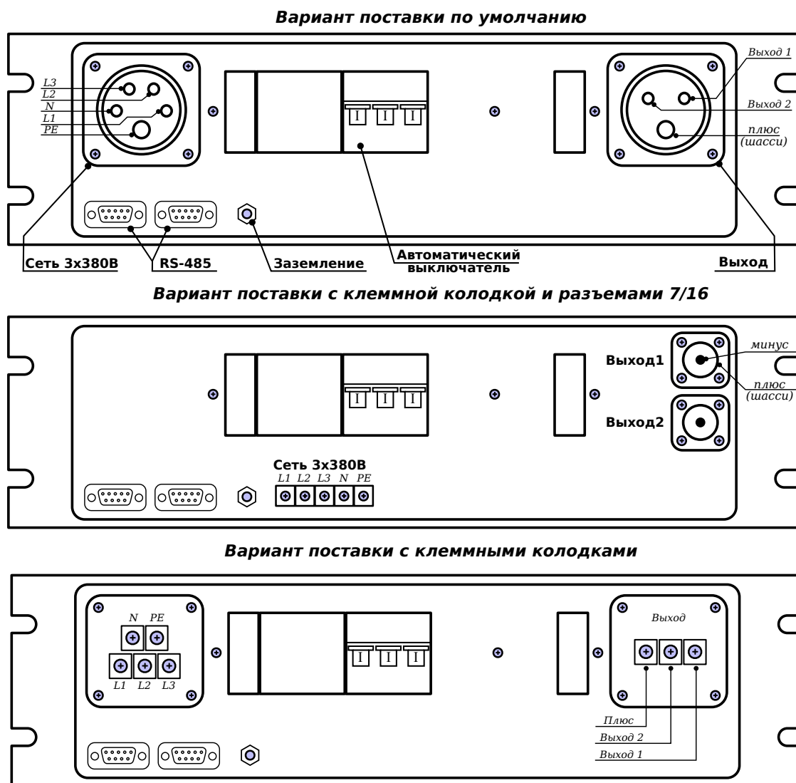
Рис. 3 — Задняя панель ИП APEL-M-10BP-1000-2.
