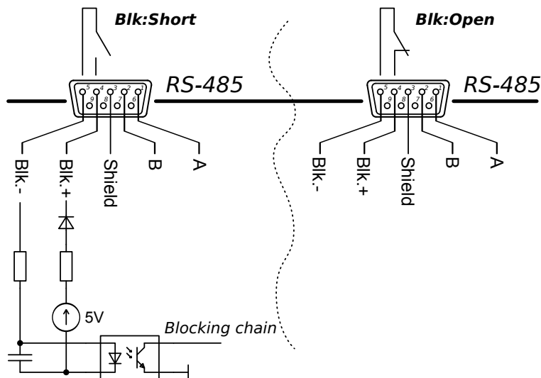
Рис. 1 — Схема цепи блокировки APEL-M-10BP-800-2.
