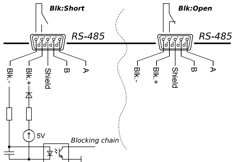
Рис. 1 — Схема цепи блокировки APEL-M-10PDC-650-1.
