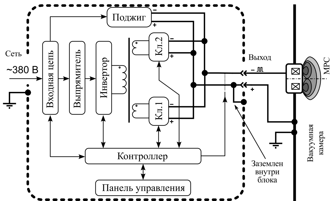
Рис. 1 — Структурная схема источника питания APEL-M-10PDC-650-1.
