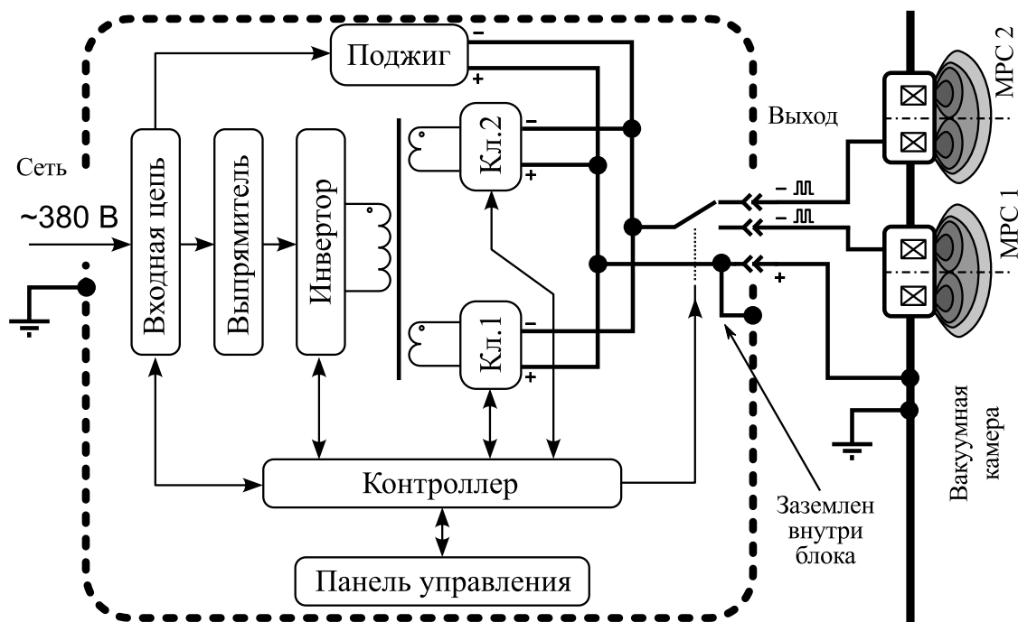
Рис. 1 — Структурная схема источника питания APEL-M-10PDC-800-2.
