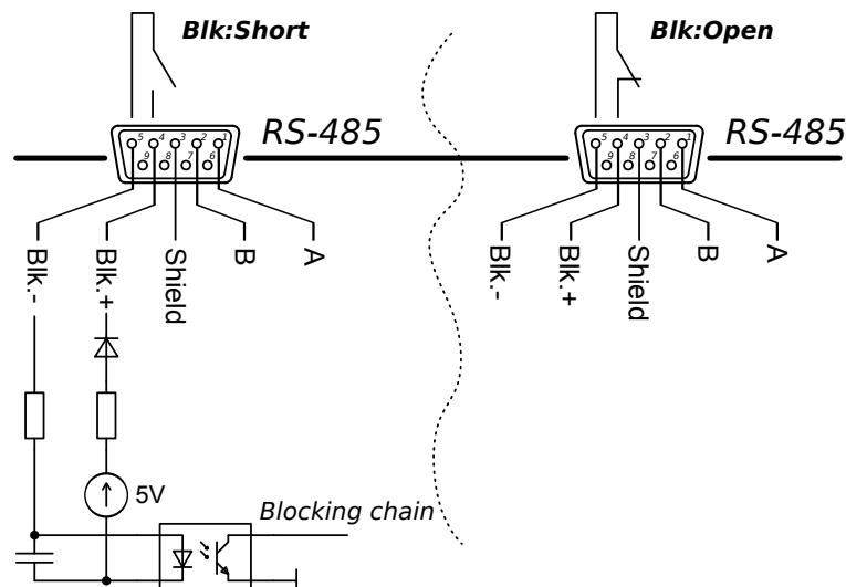
Рис. 1 — Схема цепи блокировки APEL-M-12BP-1000-1.
