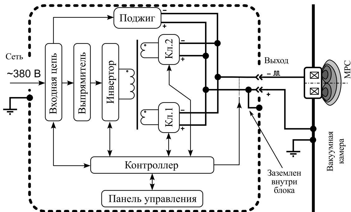
Рис. 1 — Структурная схема источника питания APEL-M-12BP-1000-1.
