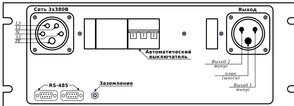
Рис. 3 — Задняя панель ИП APEL-M-12BP-800-2.
