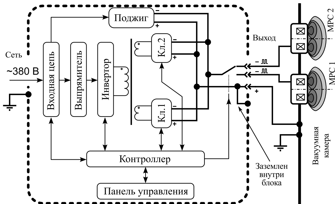
Рис. 1 — Структурная схема источника питания APEL-M-12BP-800-2.
