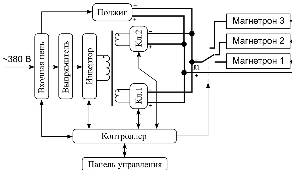
Рис. 1 — Структурная схема источника питания APEL-M-12BP-800-3.
