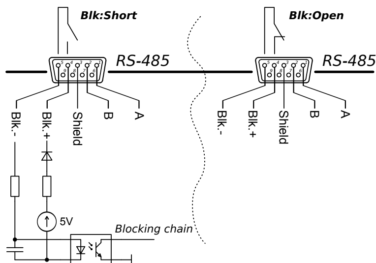
Рис. 1 — Схема цепи блокировки APEL-M-12BP-800-3.
