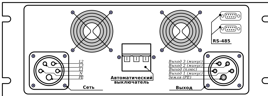
Рис. 3 — Задняя панель ИП APEL-M-12BP-800-3.
