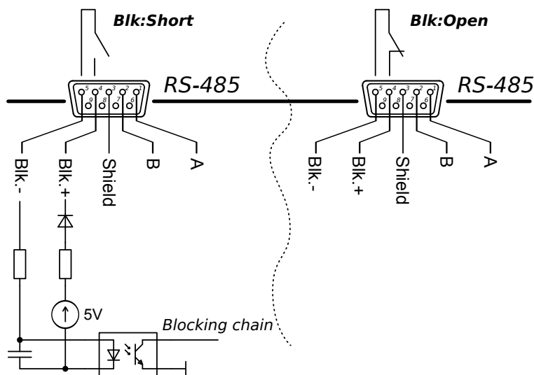
Рис. 1 — Схема цепи блокировки APEL-M-5PDC-1000-1.
