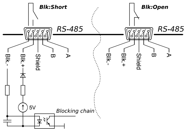
Рис. 1 — Схема цепи блокировки АРЕL-SB-10BP-800-1.
