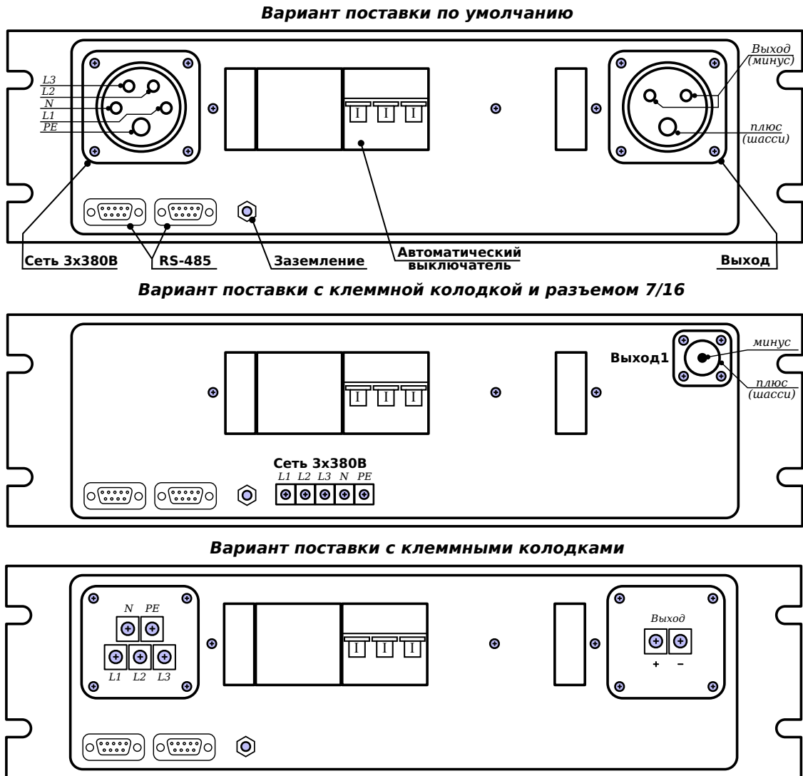
Рис. 3 — Задняя панель ИП APEL-SB-10BP-800-1.
