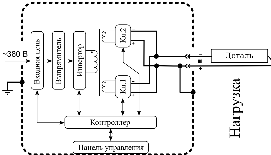
Рис. 1 — Структурная схема источника питания APEL-SB-10BP-800-1.
