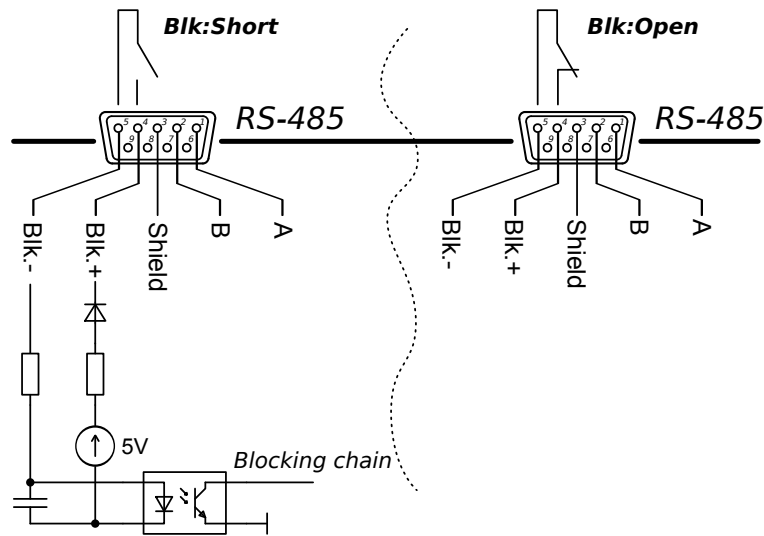
Рис. 1 — Схема цепи блокировки APEL-SB-12BP-1500-1.
