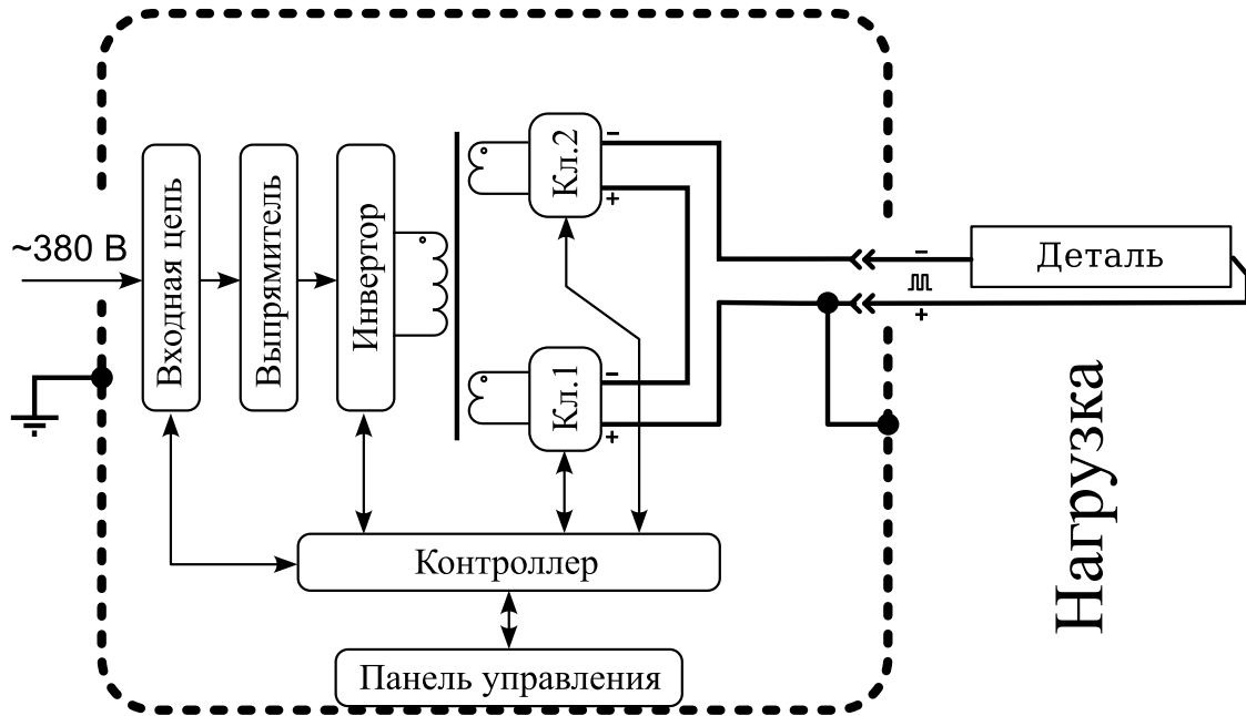
Рис. 1 — Структурная схема источника питания APEL-SB-12BP-1500-1.
