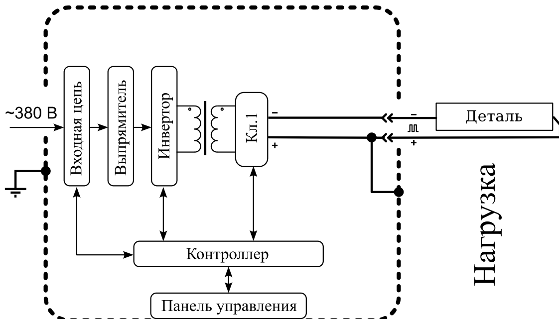
Рис. 1 — Структурная схема источника питания APEL-SB-3PDC-650-1.
