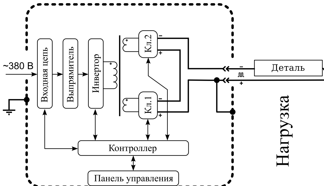
Рис. 1 — Структурная схема источника питания APEL-SB-5PDC-1500-1.
