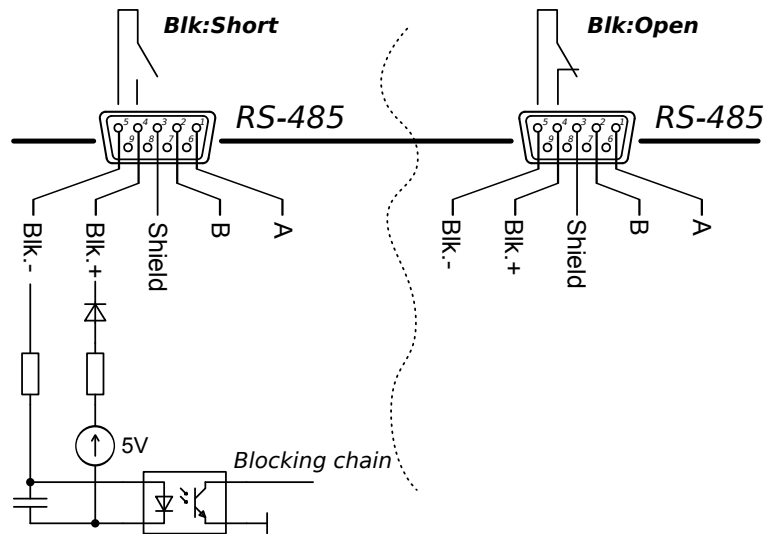
Рис. 1 — Схема цепи блокировки APEL-SB-5PDC-1500-1.
