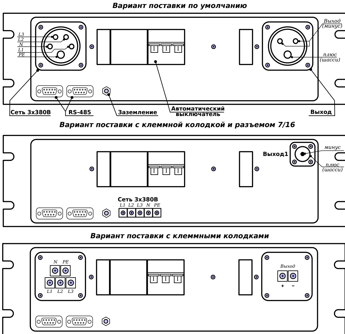
Рис. 3 — Задняя панель ИП APEL-SB-5PDC-1500-1.
