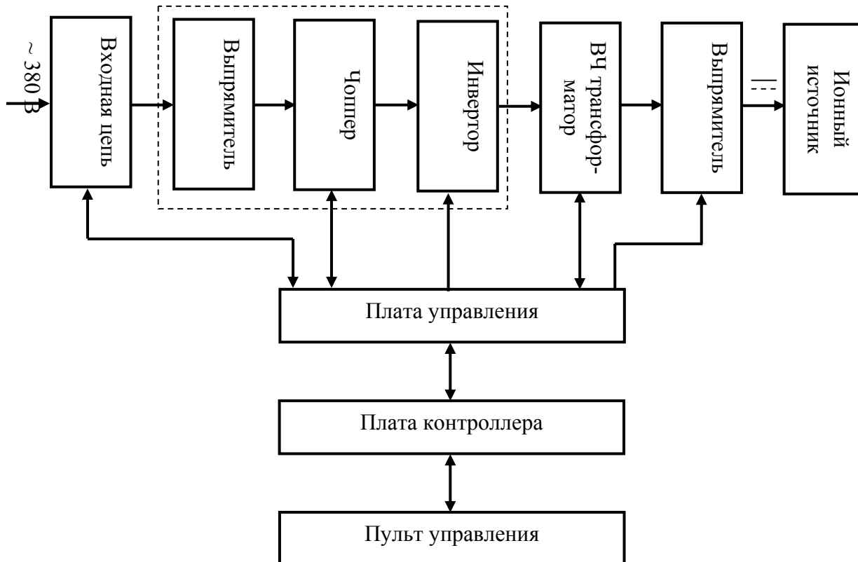
Рис. 1. Блок-схема источника питания APEL-IS-5000.
