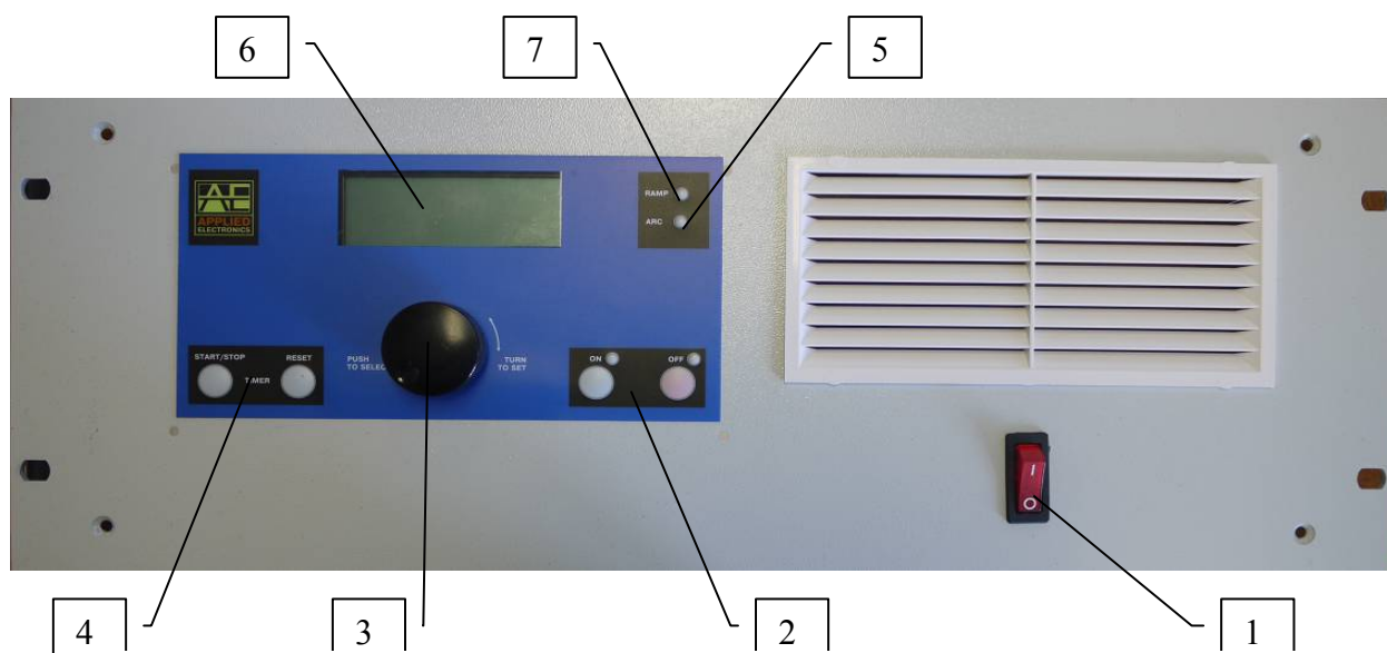
Рис. 2. Расположение органов управления на передней панели источника питания APEL-IS-5000
