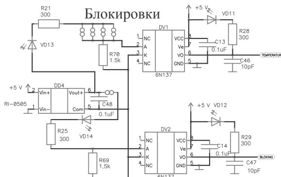
Рис. 11 Схема организации блокировок источника
