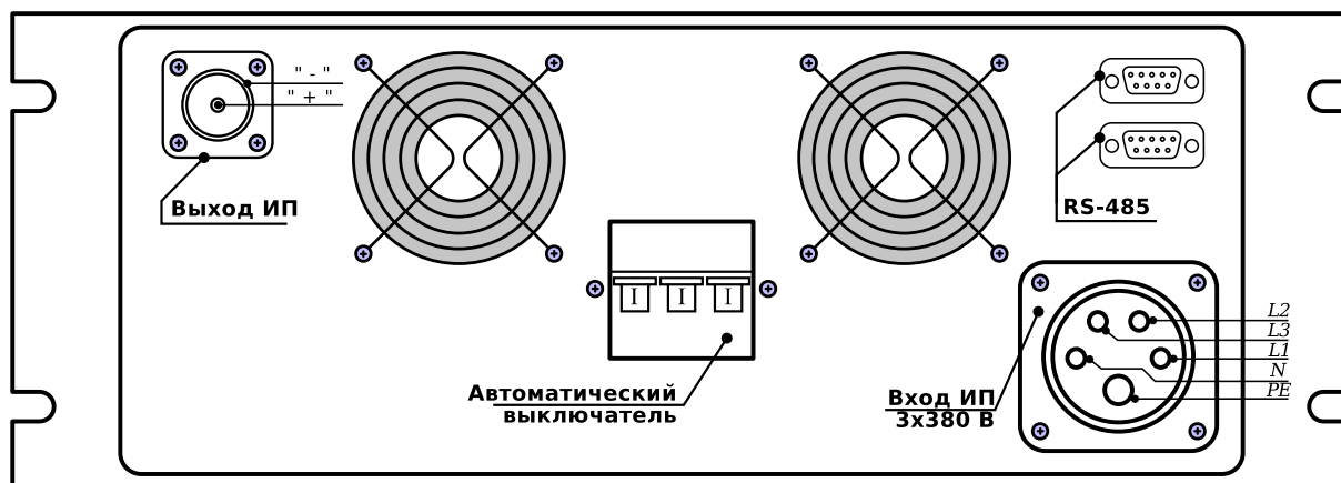
Рис. 4 — Задняя панель ИП APEL-IS-3500.
