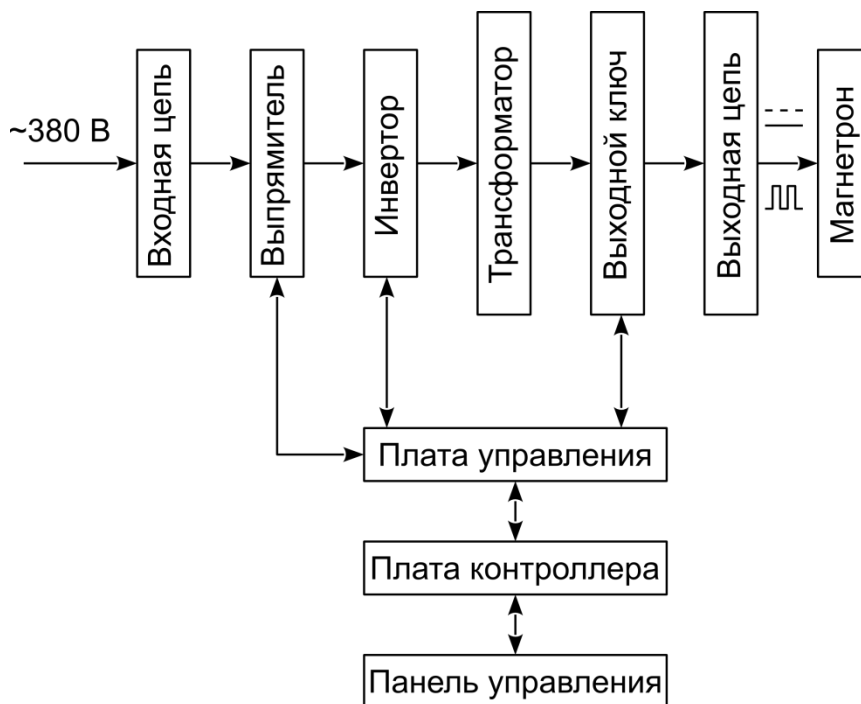
Рис. 1 — Структурная схема ИП APEL-M-5PDC-650-2.
