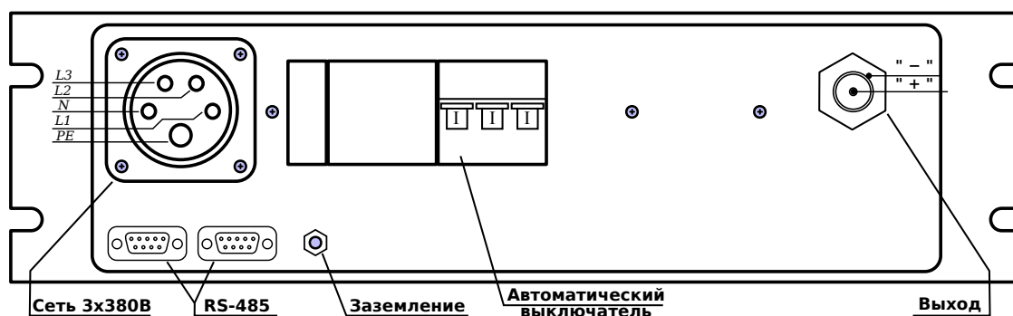
Рис. 3 — Задняя панель ИП APEL-IS-2000.
