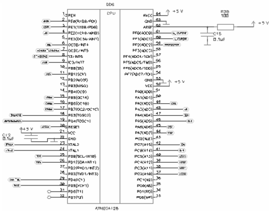
Рис. 5 Микроконтроллер Atmega128. Формирование сигналов: Импульсные выходы
