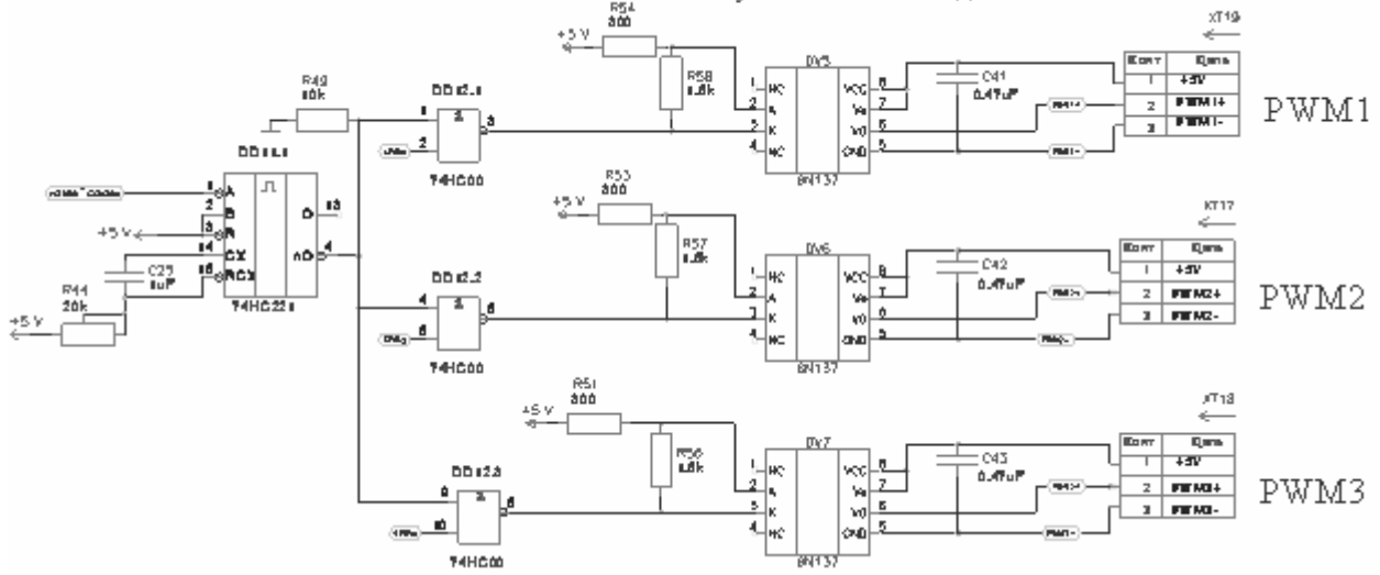
Рис. 5 Микроконтроллер Atmega128. Формирование сигналов: Импульсные выходы
